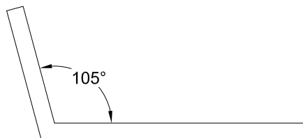
BÄRARMS VINKEL 700.05
